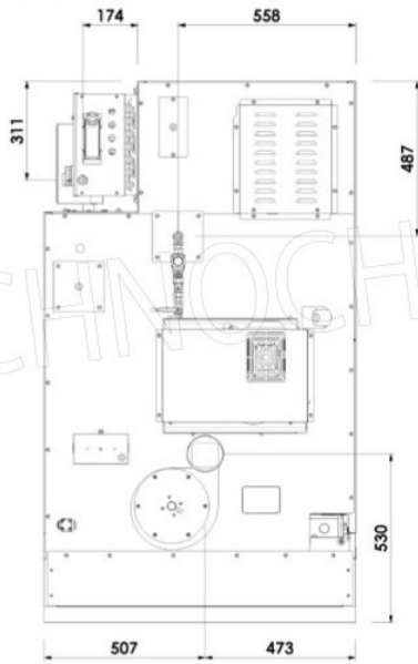
VISTA SUPERIORE
