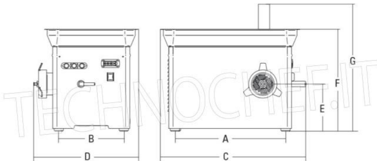
Dimensioni mm
